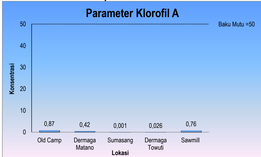
Gambar 4.8 Hasil Uji Parameter Klorofil A Untuk Air Danau
