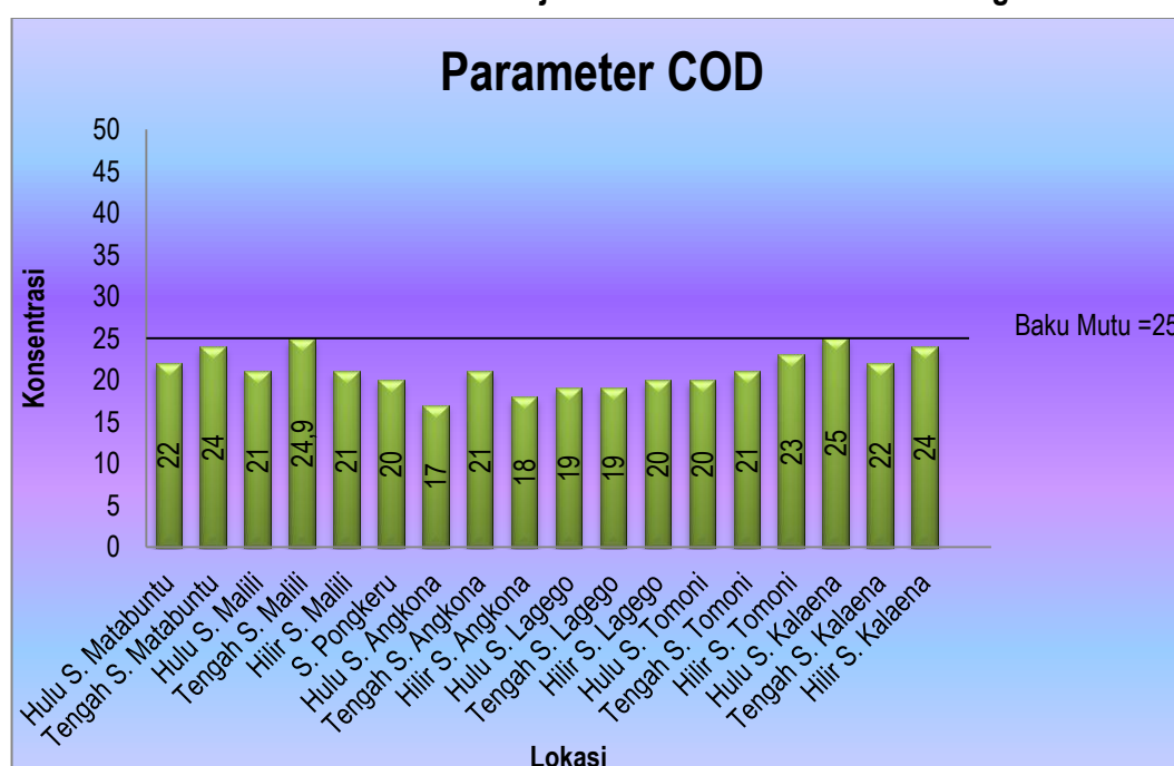
Gambar 4.14 Hasil Uji Parameter COD Untuk Air Sungai
