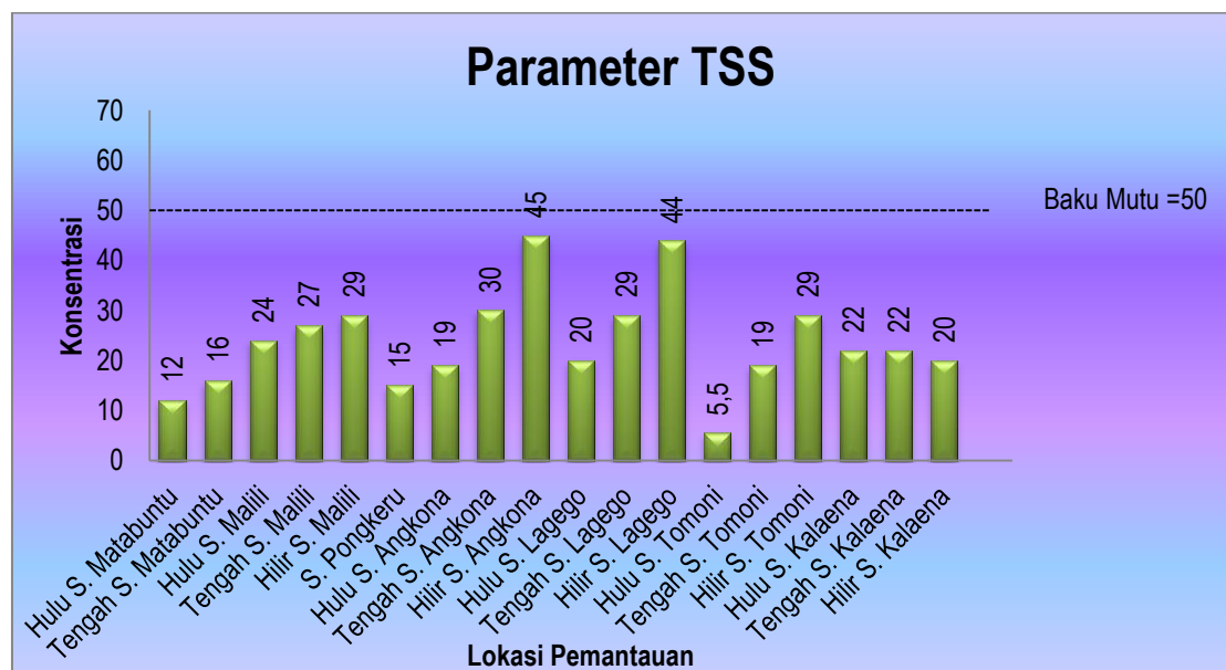
Gambar 4.12 Hasil Uji Parameter TSS Untuk Air Sungai
