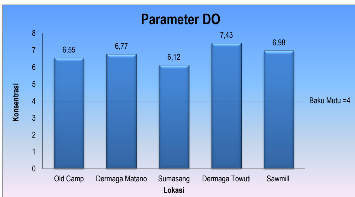
Gambar 4.3 Hasil Uji Parameter DO Untuk Air Danau
