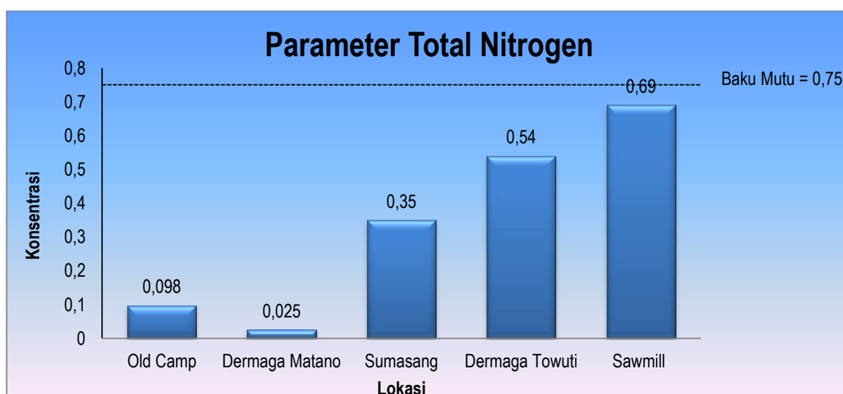
Gambar 4.6 Hasil Uji Parameter Total Nitrogen Untuk Air Danau
