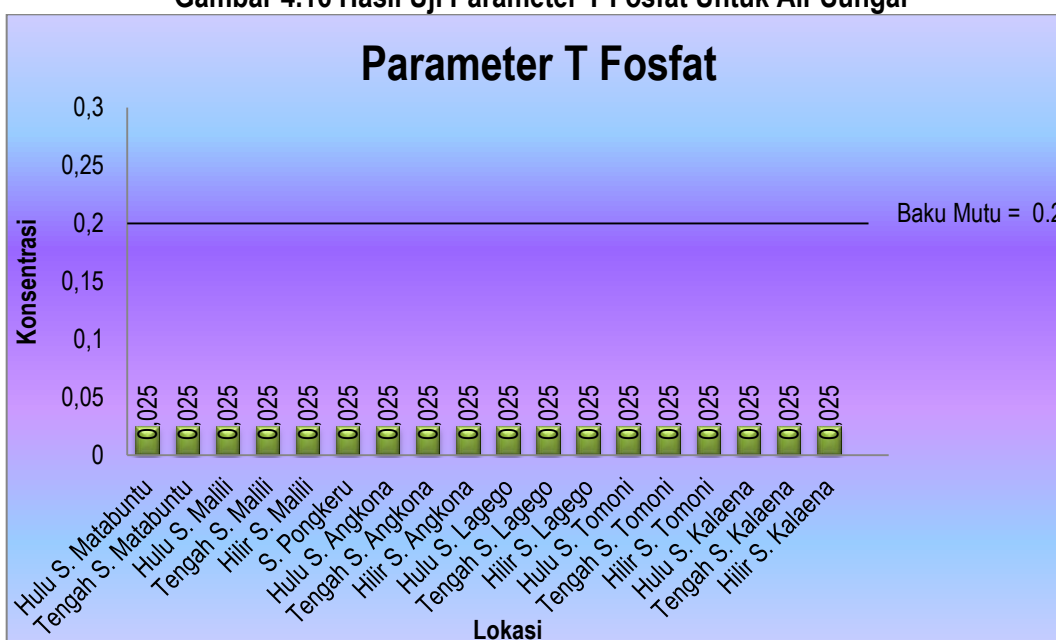
Gambar 4.16 Hasil Uji Parameter T Fosfat Untuk Air Sungai
