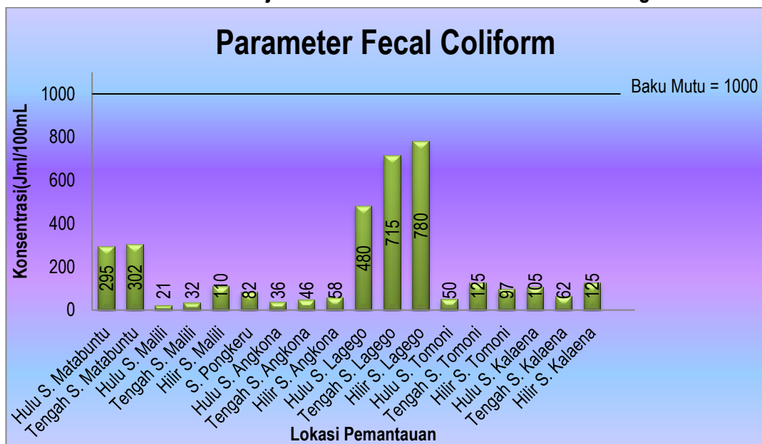
Gambar 4.18 Hasil Uji Parameter Fecal Coliform Untuk Air Sungai
