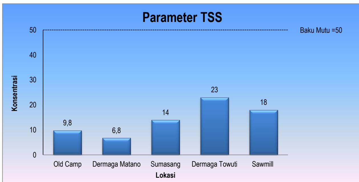
Gambar 4.2 Hasil Uji Parameter TSS Untuk Air Danau
