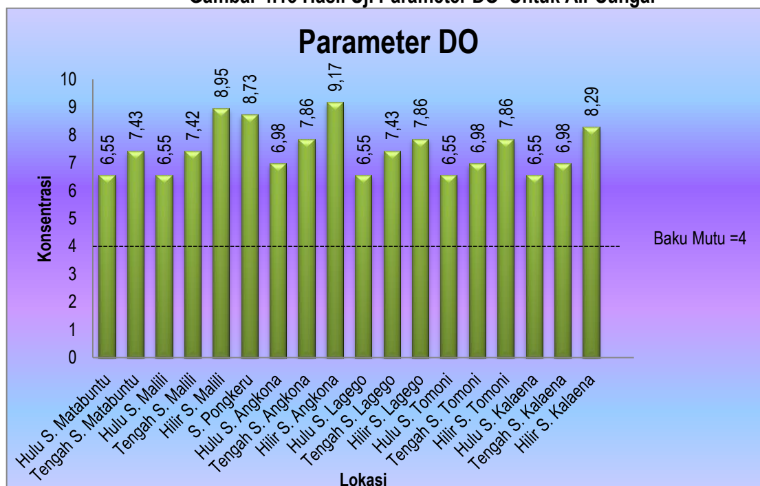
Gambar 4.13 Hasil Uji Parameter DO Untuk Air Sungai
