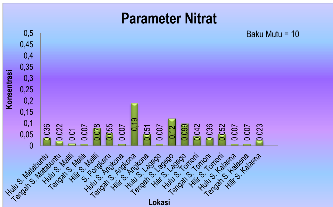
Gambar 4.17 Hasil Uji Parameter Nitrat Untuk Air Sungai
