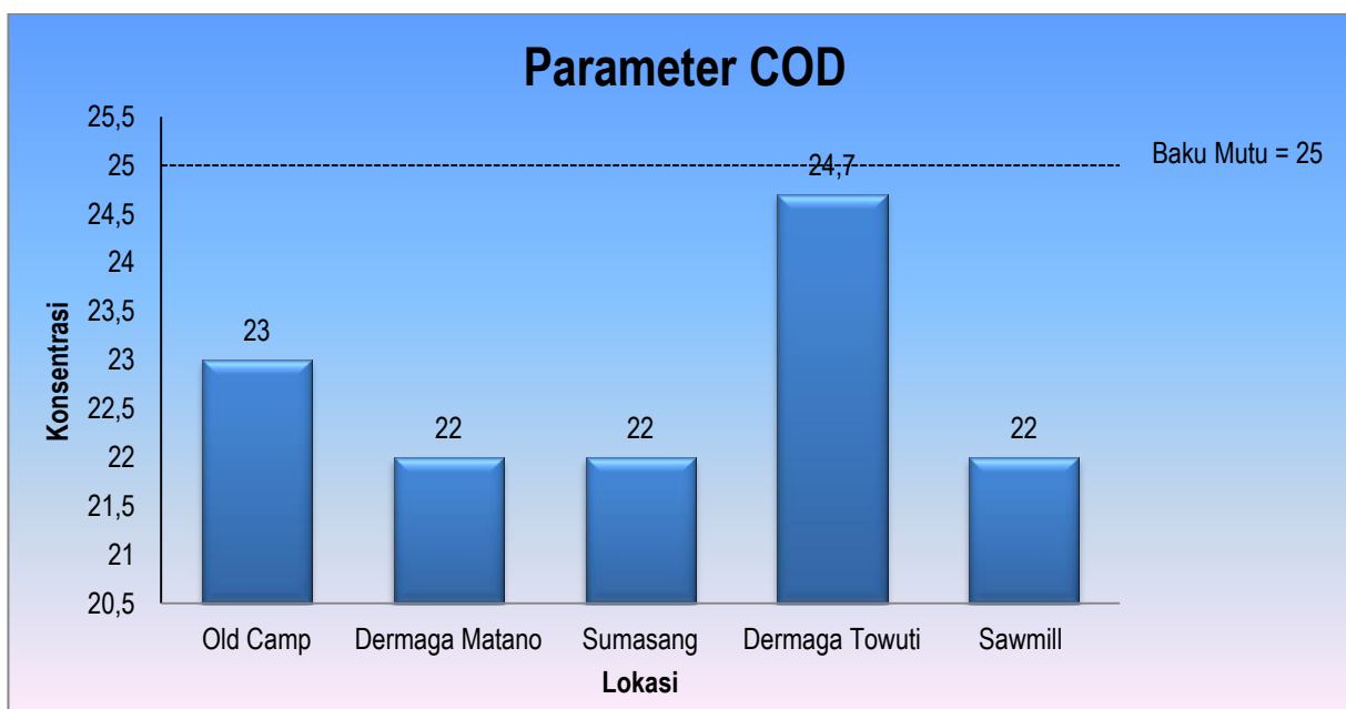
Gambar 4.4 Hasil Uji Parameter COD Untuk Air Danau
