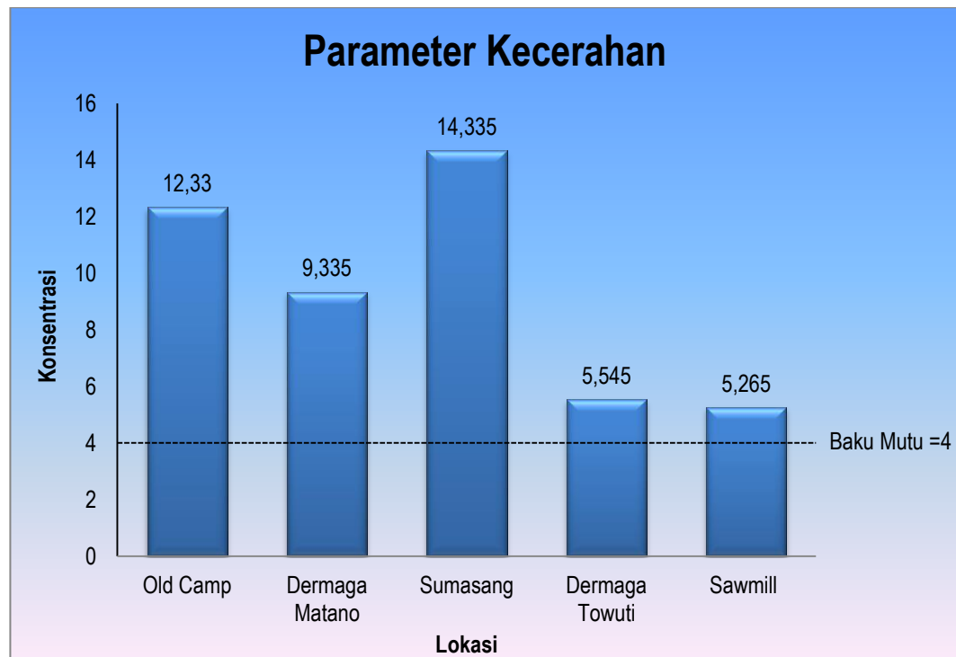
Gambar 4.9 Hasil Uji Parameter Kecerahan Untuk Air Danau
