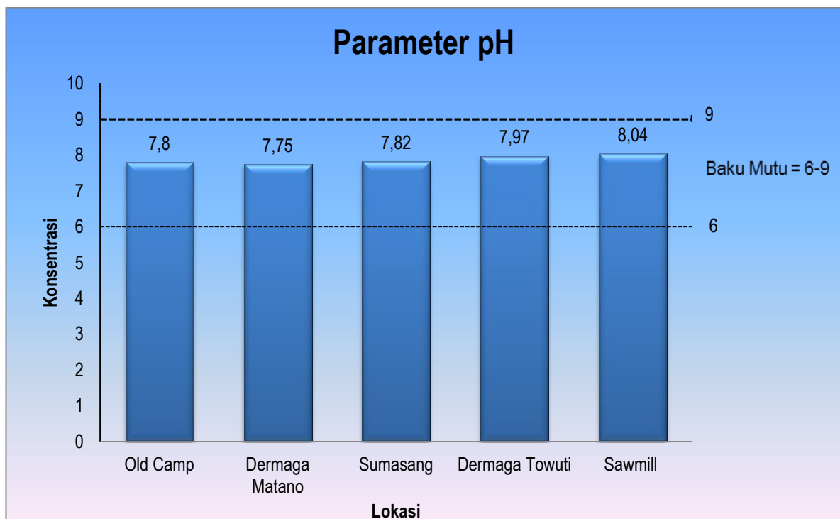
Gambar 4.1 Hasil Uji Parameter pH Untuk Air Danau
