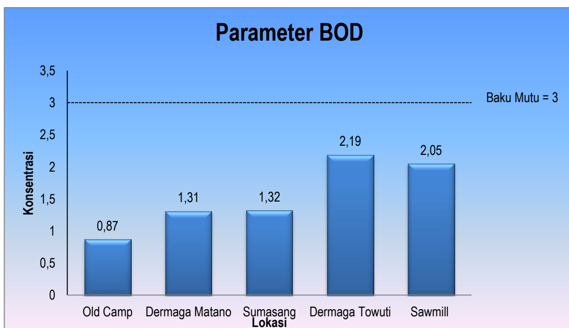
Gambar 4.5 Hasil Uji Parameter BOD Untuk Air Danau
