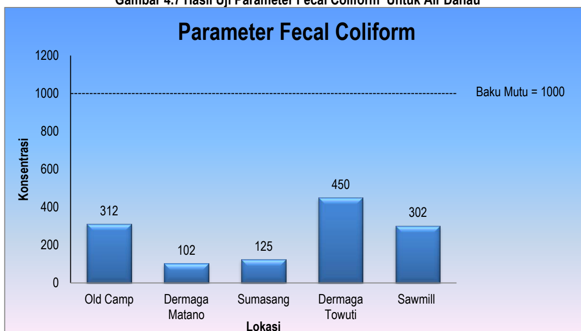
Gambar 4.7 Hasil Uji Parameter Fecal Coliform Untuk Air Danau
