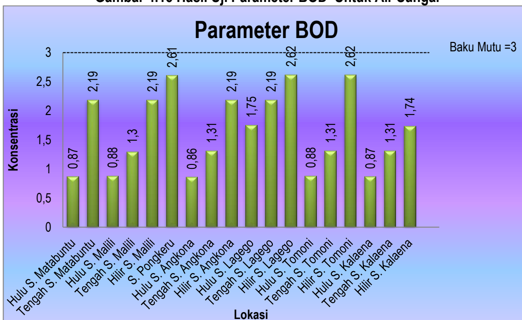
Gambar 4.15 Hasil Uji Parameter BOD Untuk Air Sungai
