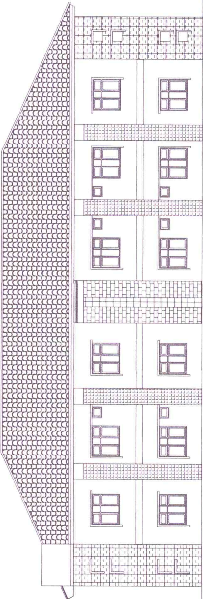
VIEW 1 EKSTING (TAMPAK SAMPING KANAN) EKS Skala 1 : 150
