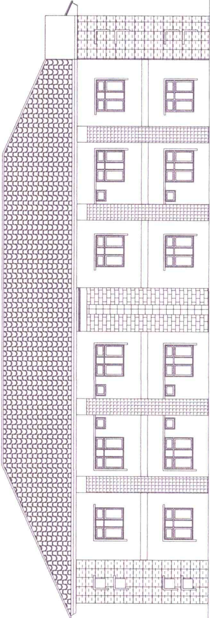
VIEW 2 EKSTING (TAMPAK SAMPING KIRI) EKS Skala 1 : 150
