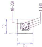
DETAIL KOLOM PRAKTIS
