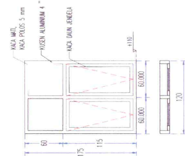
JENDELA J1
